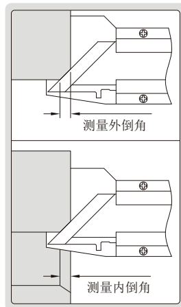
测量倒角尺寸
