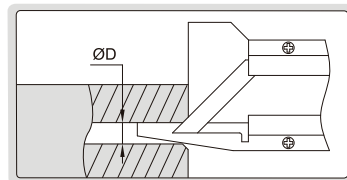
测量内孔时, 内孔直径>ØD
